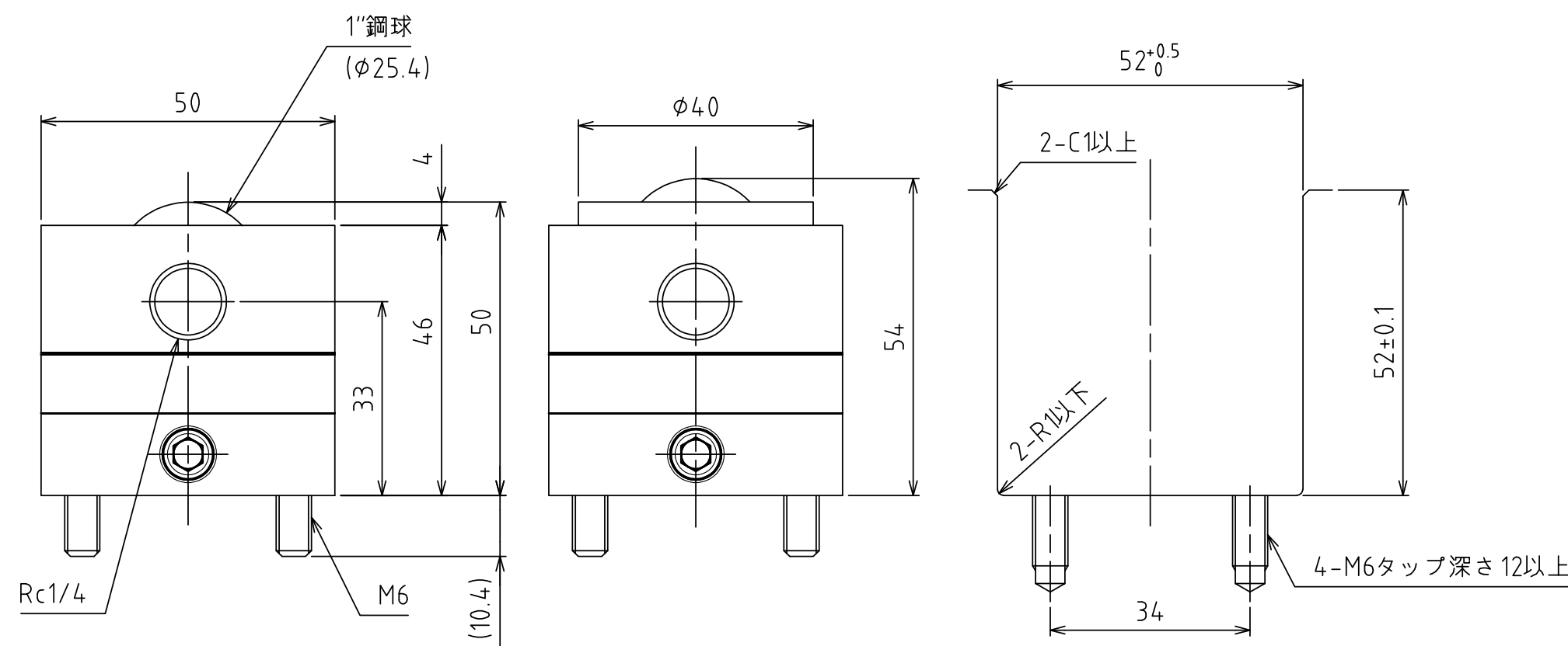
A矢視図
