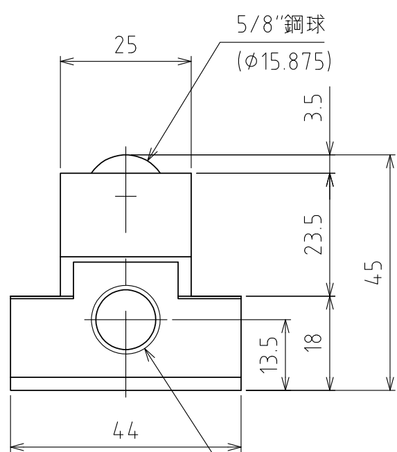
A矢視図
