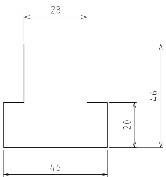
T溝寸法
