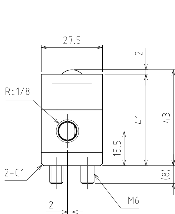
A矢視図
