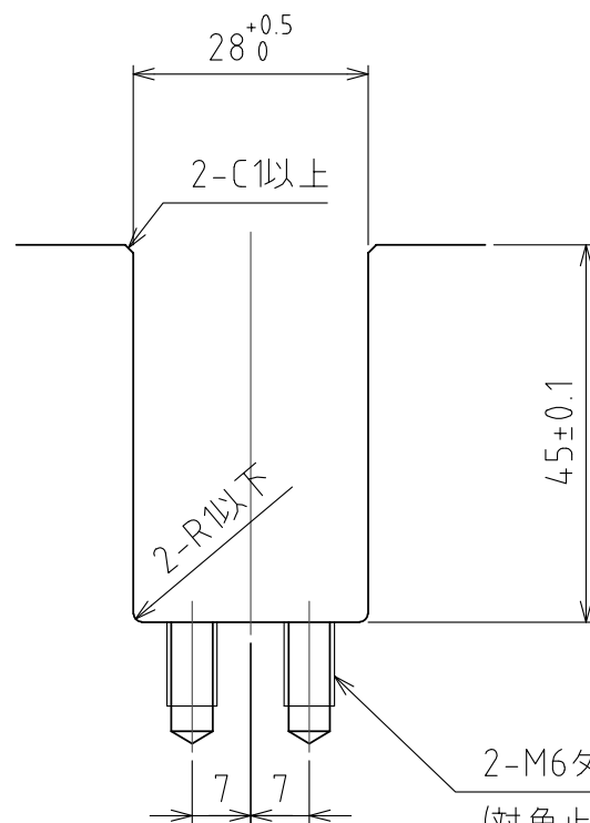
推奨溝寸法
