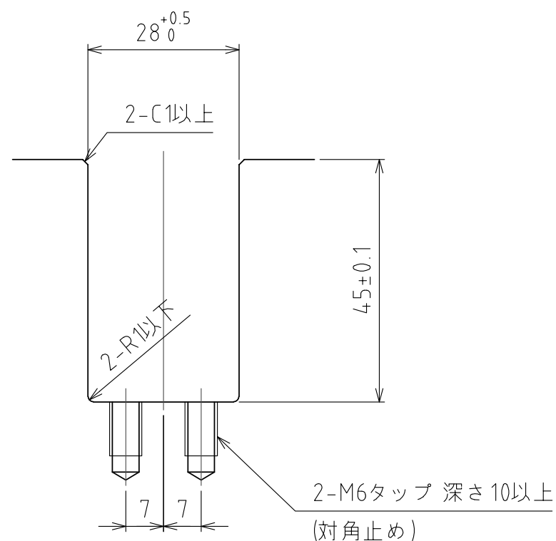
推奨溝寸法
