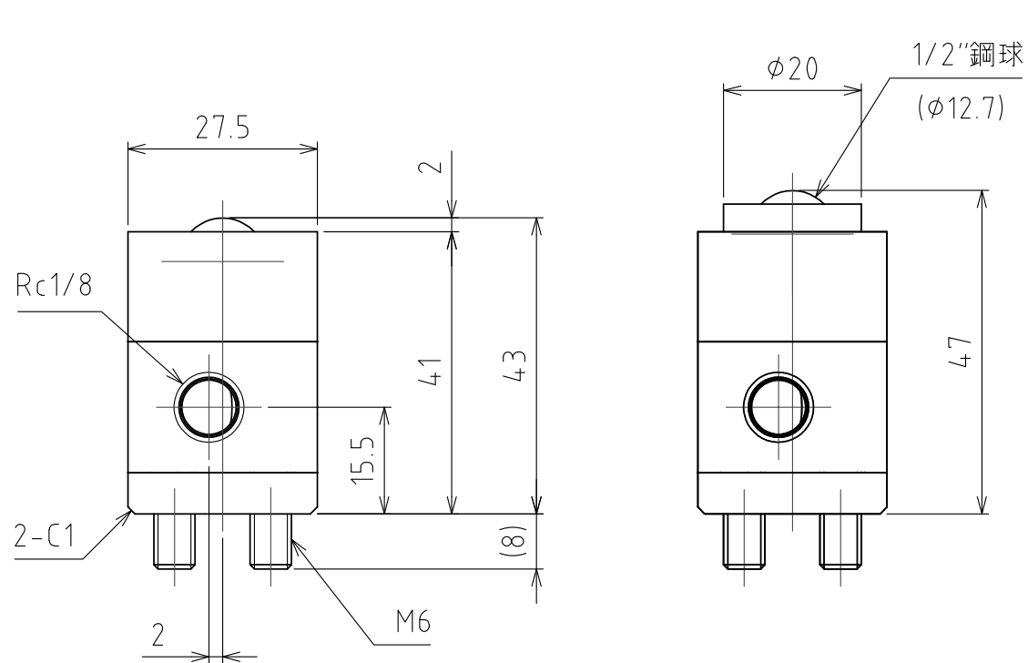
A矢視図
