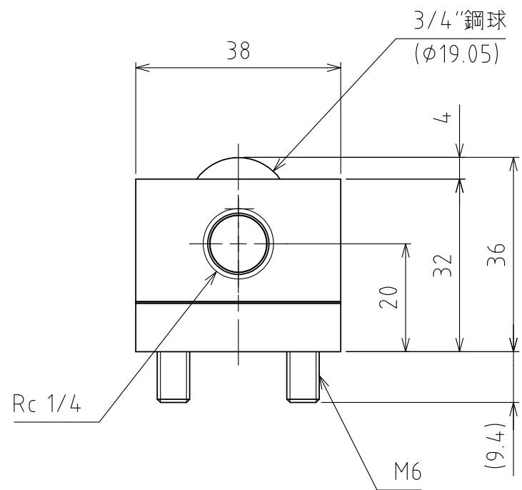
A矢視図
