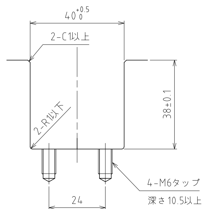
推奨溝寸法
