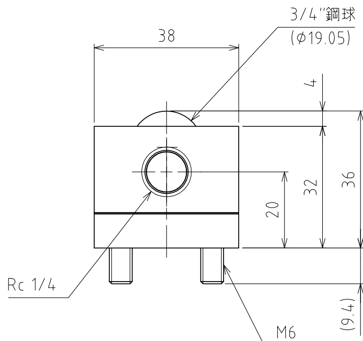
A矢視図
