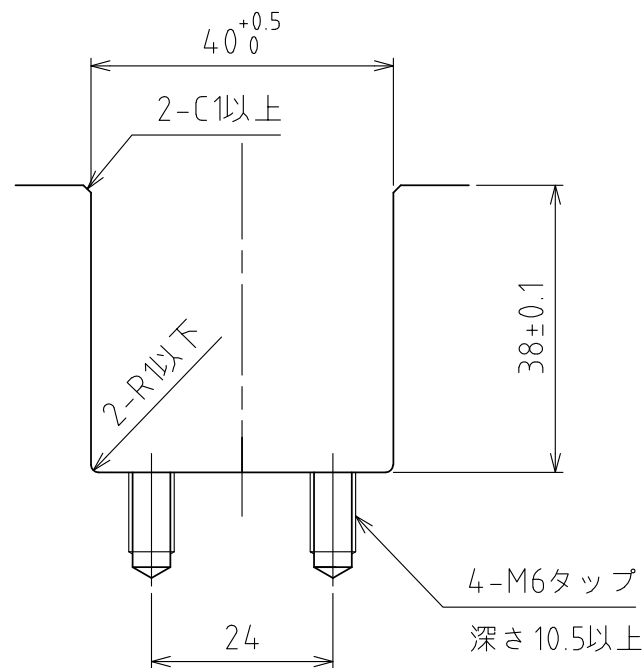
推奨溝寸法
