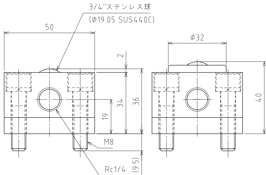
A矢視図
