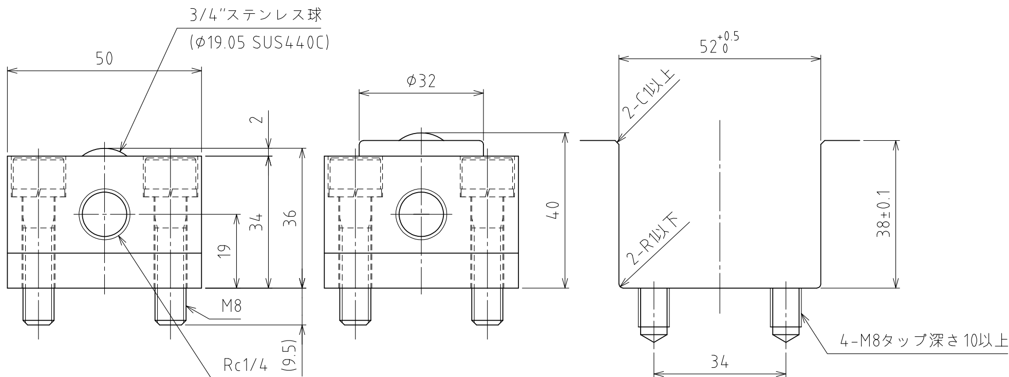
A矢視図
