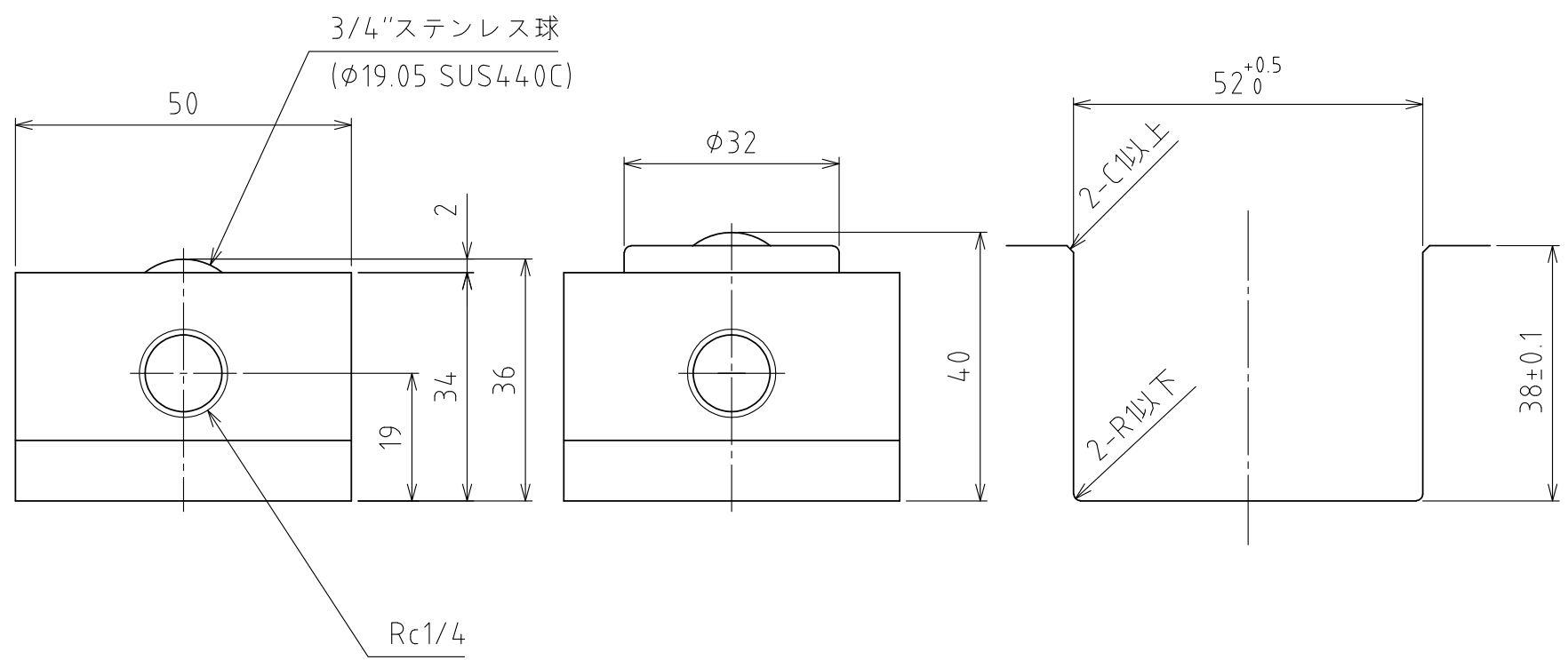
A矢視図
