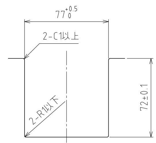
推奨溝寸法
