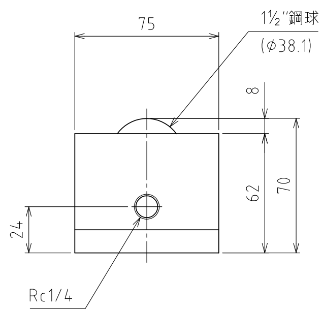
A矢視図
