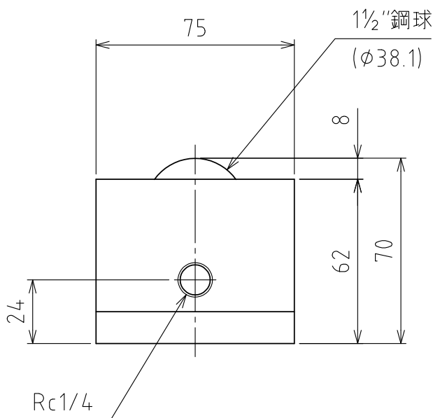
A矢視図
