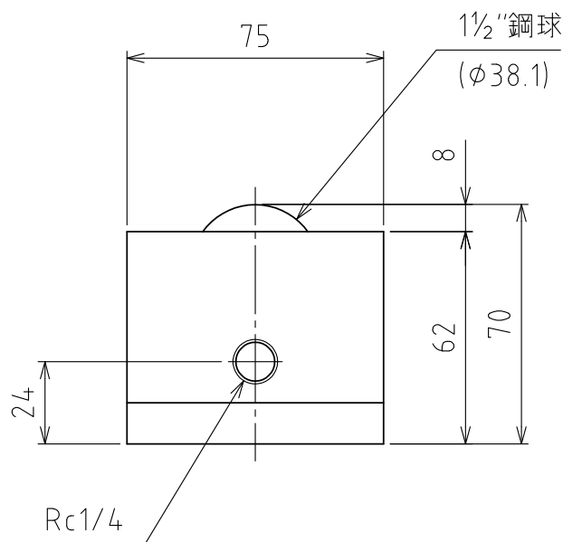
A矢視図
