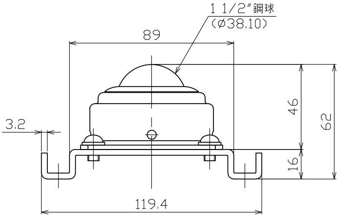
A矢視図 (SCALE 1:3)
