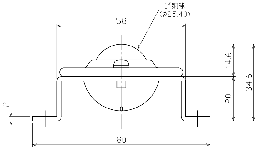
A矢視図 (SCALE 1:1)
