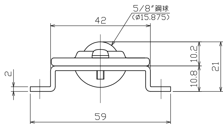
A矢視図 (SCALE 1:1)
