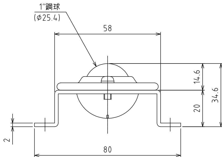
A矢視図
