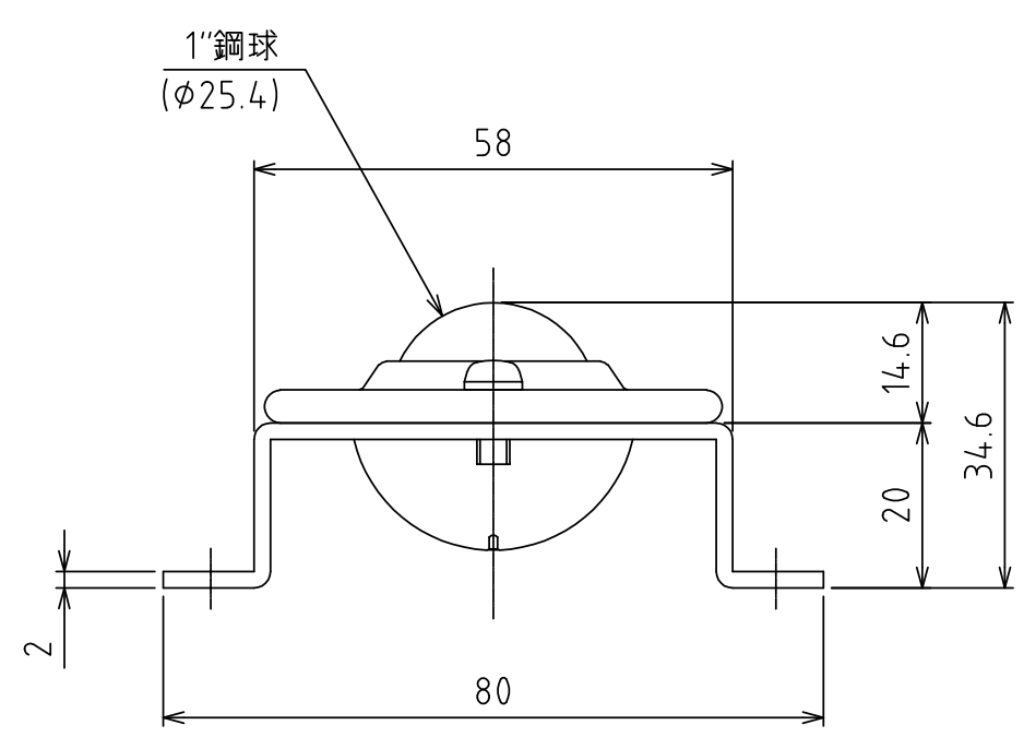
A矢視図 (尺度 1:1)
