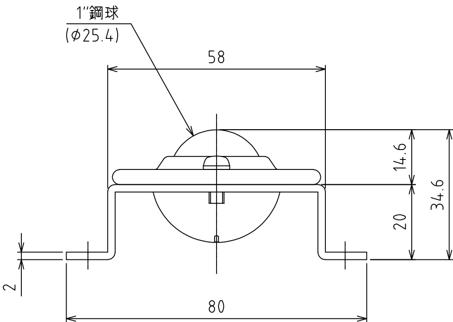
A矢視図
