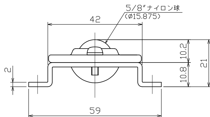
A矢視図 (SCALE 1:1)
