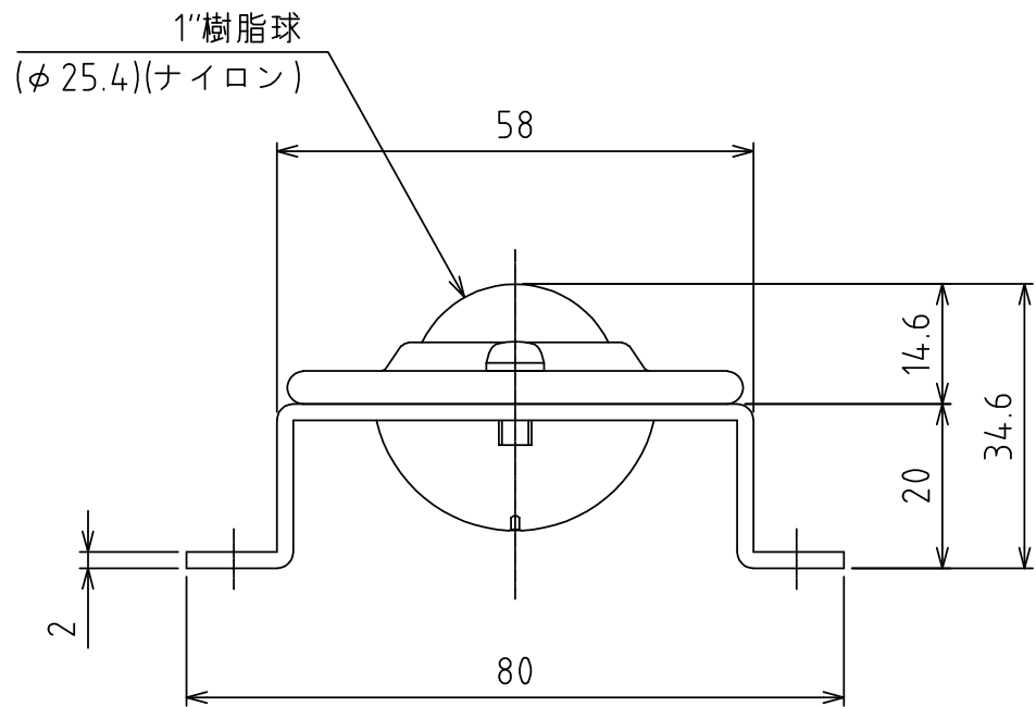
A矢視図
