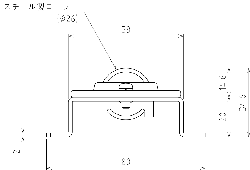
A矢視図
