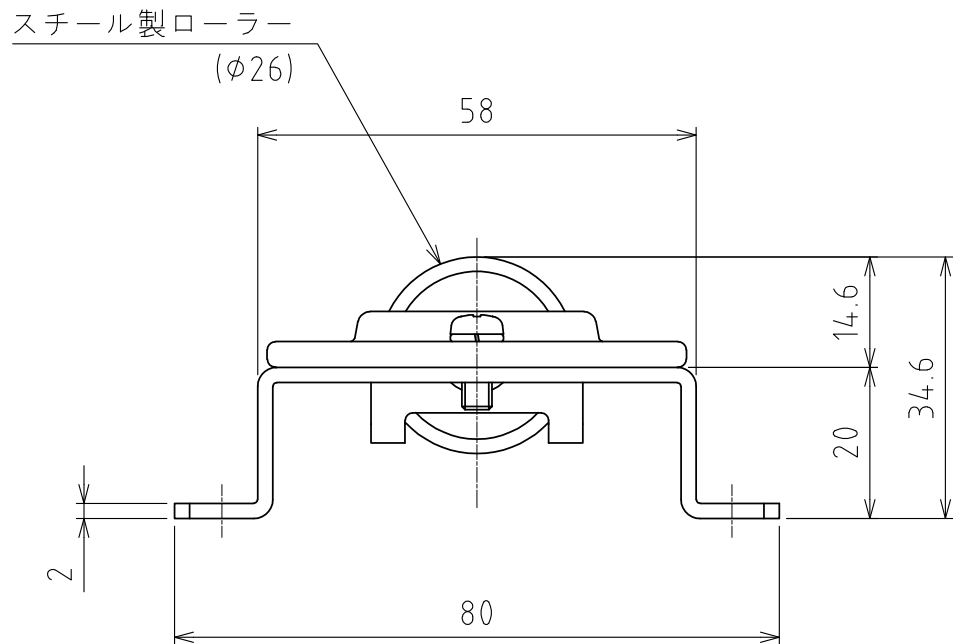
A矢視図
