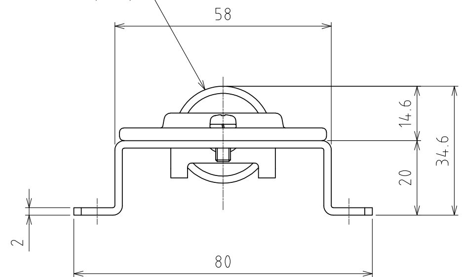
A矢視図 (尺度 1:1)
