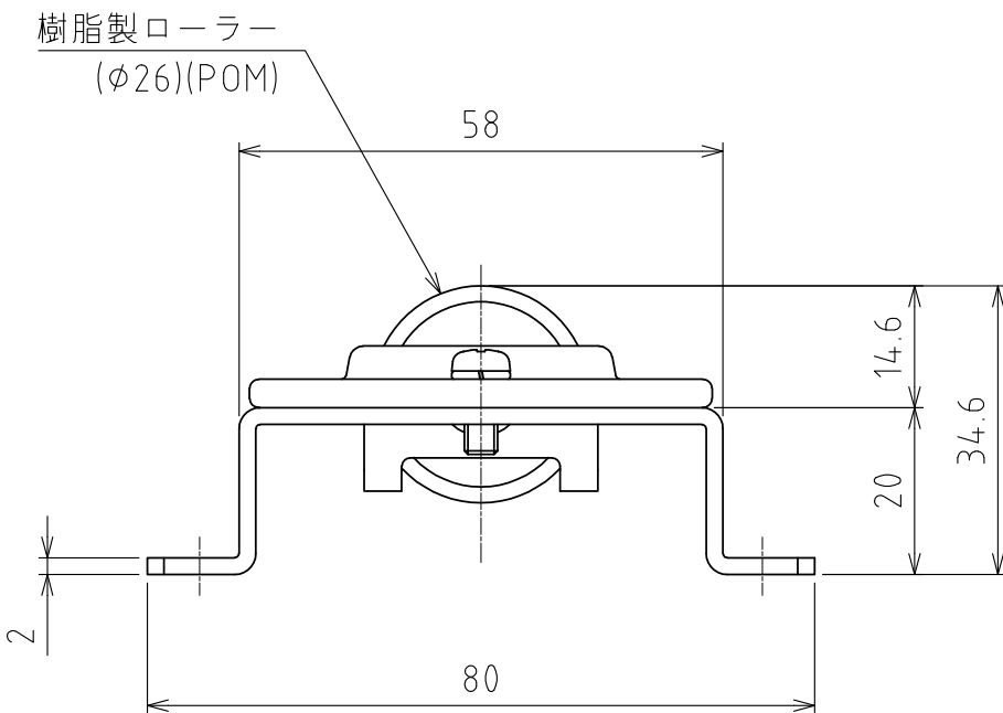
A矢視図
