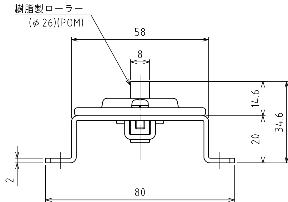
A矢視図
