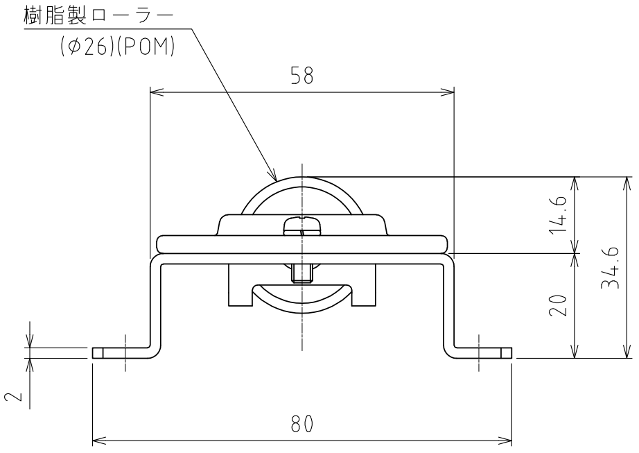
A矢視図 (尺度 1:1)
