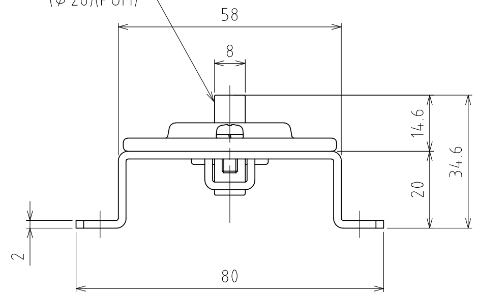
A矢視図 (尺度 1:1)
