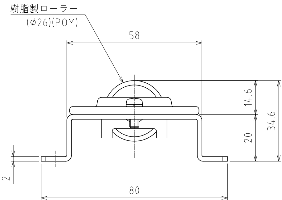
A矢視図
