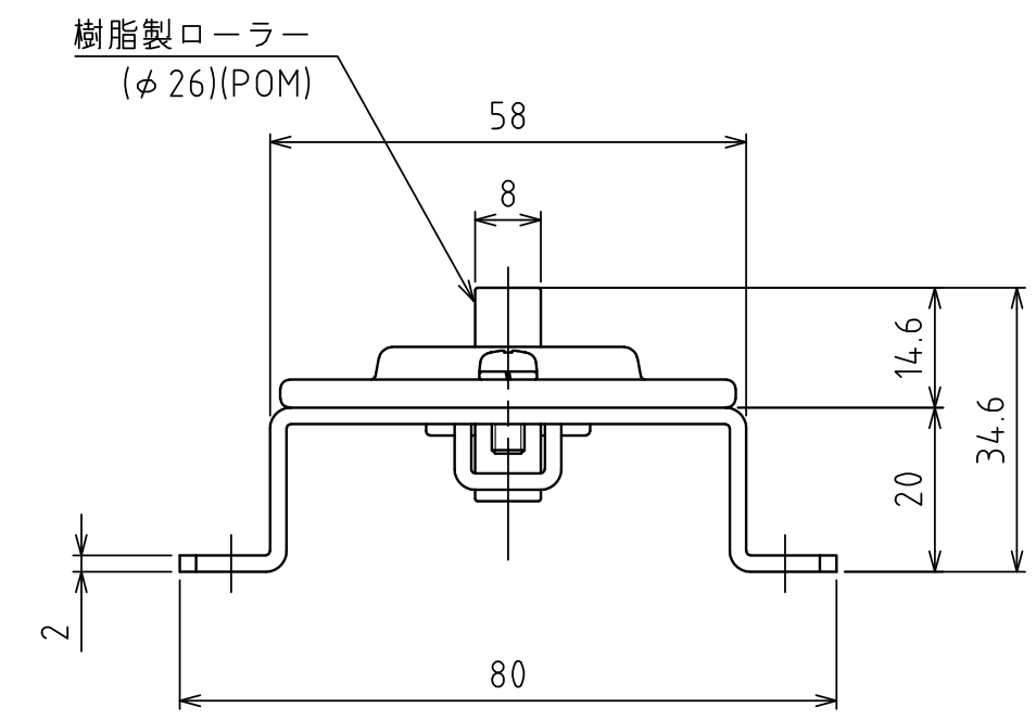
A矢視図 (尺度 1:1)
