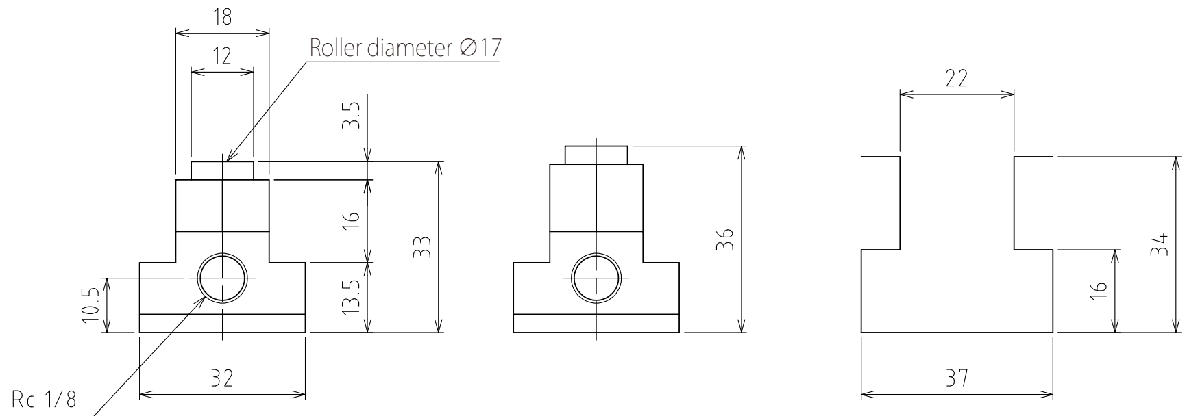
Rising (stroke 3mm) (Scale 1:1)
