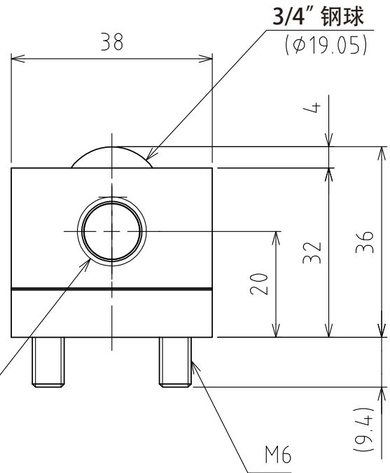
A视图
