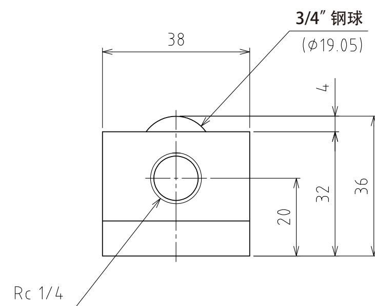
A视图
