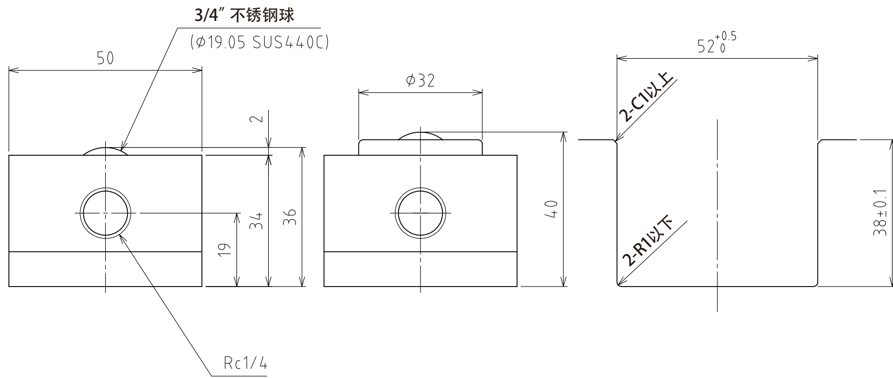
A视图
