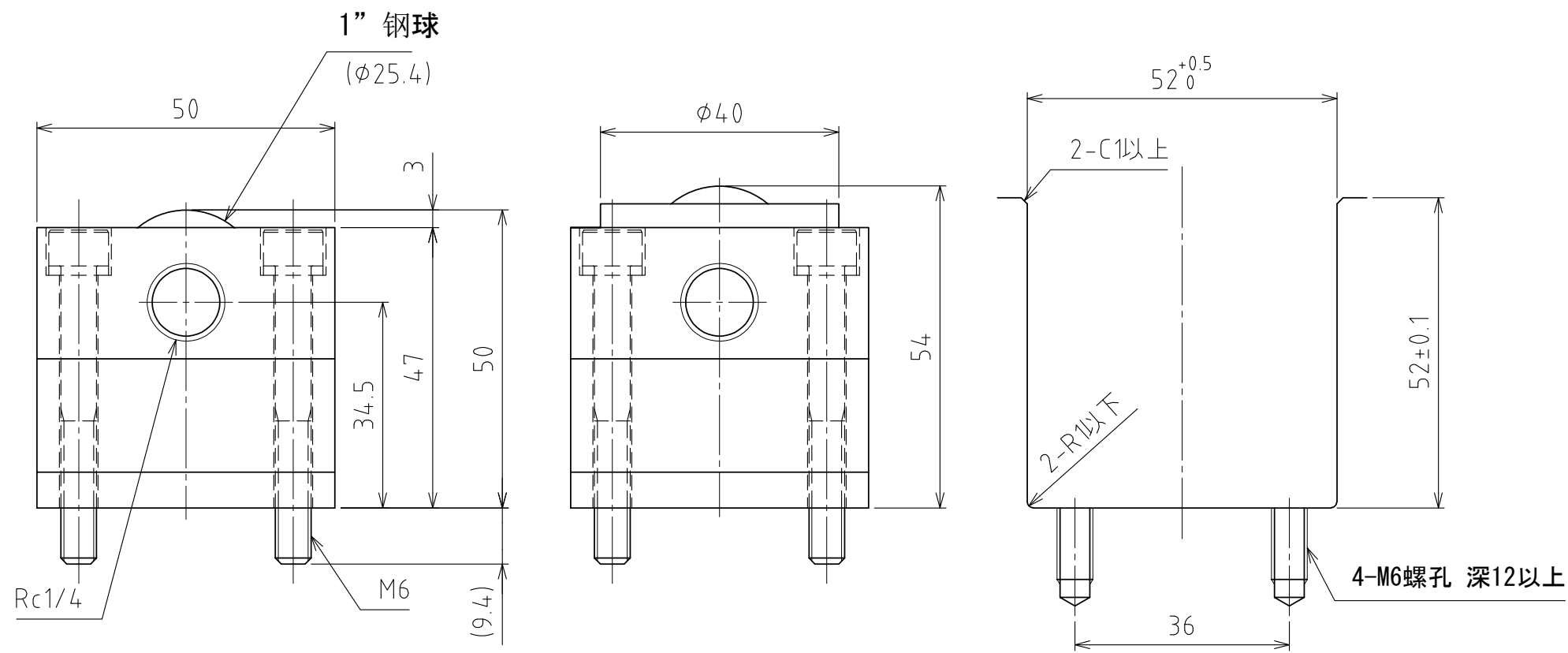
上浮时 (行程4mm) (尺度 1:1)
