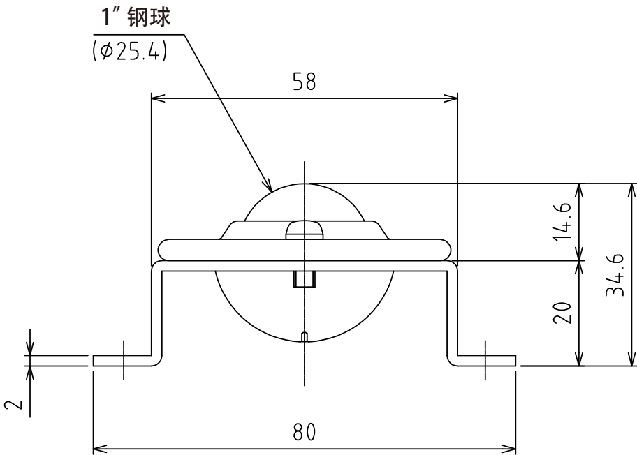
A视图 (尺度 1:1)
