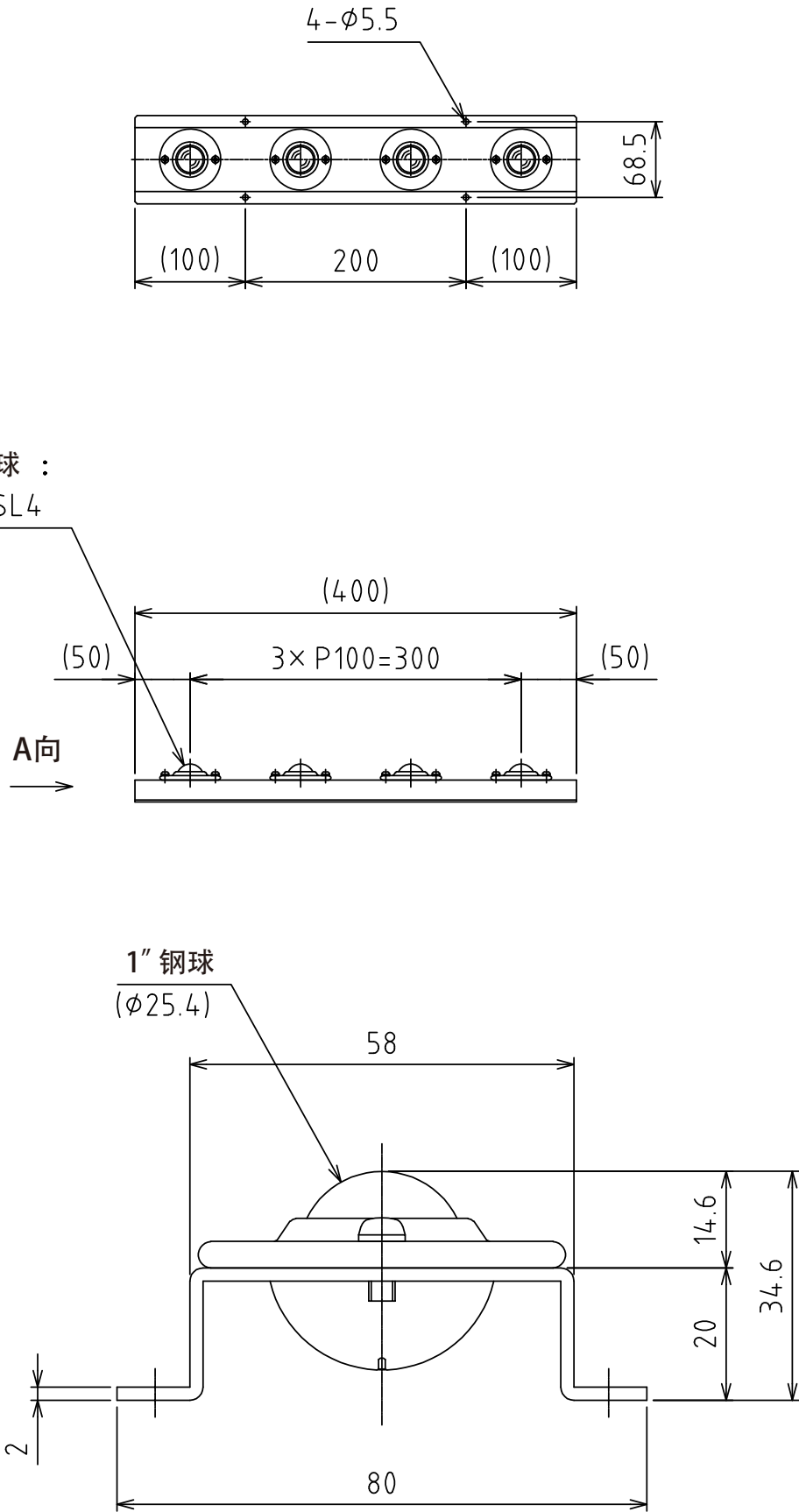
A视图 (尺度 1:1)
