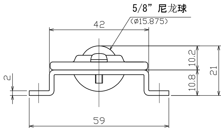
A视图 (尺度 1 : 1)
