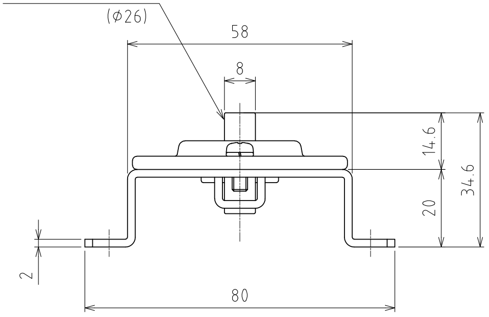
A视图 (尺度 1:1)
