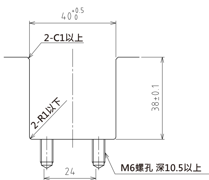
推薦的凹槽尺寸
