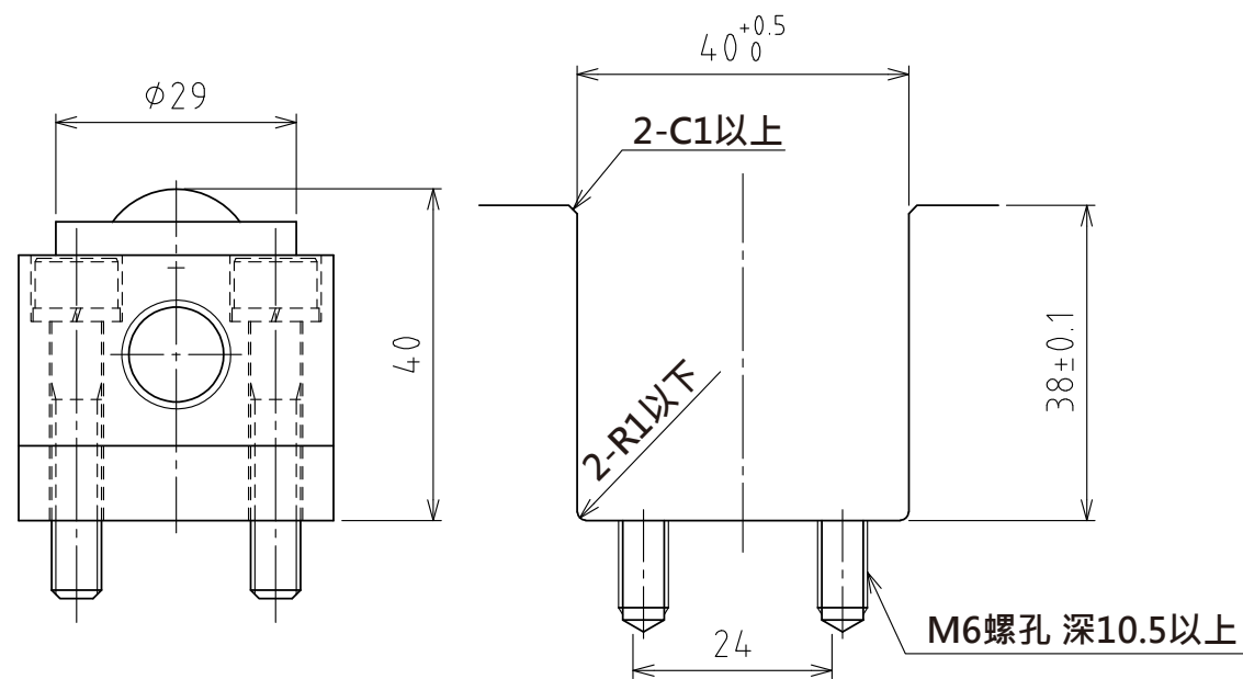
上浮時 (行程4mm) (尺度 1:1)
