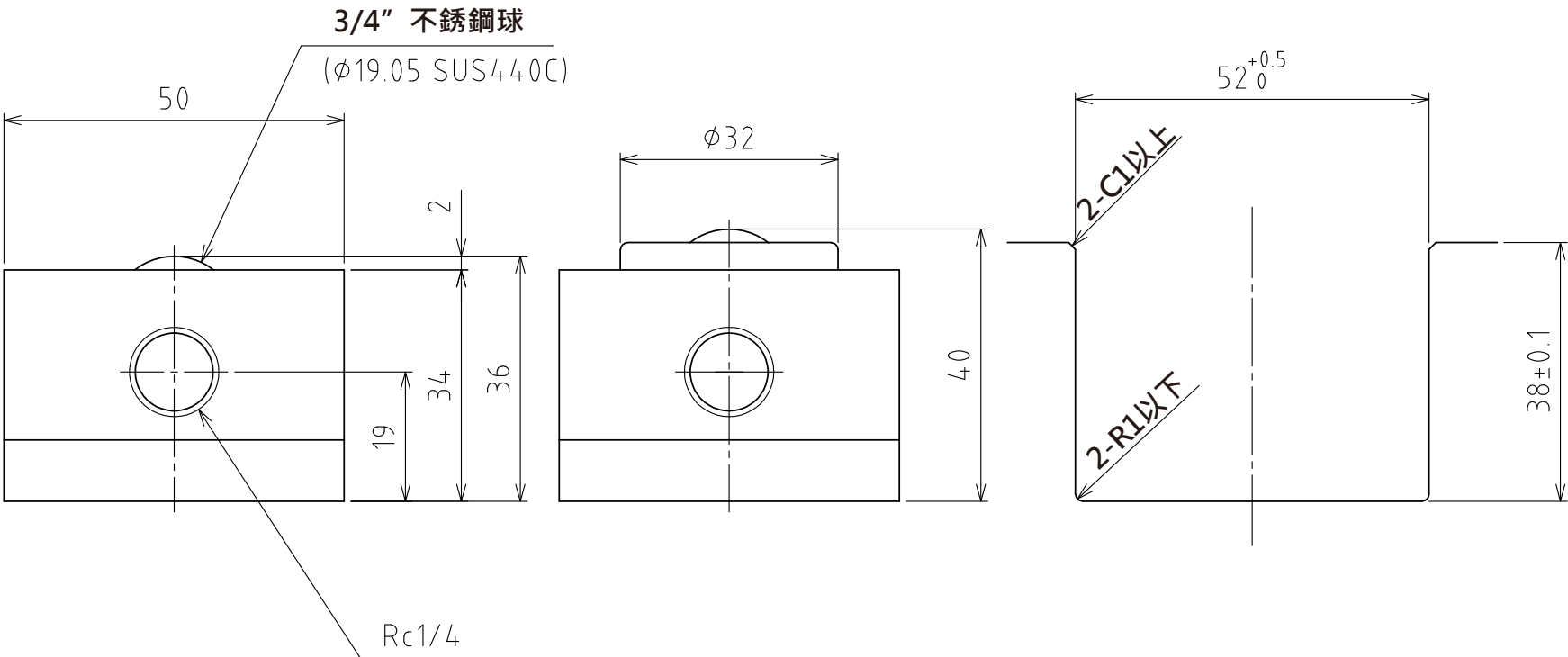
A視圖
