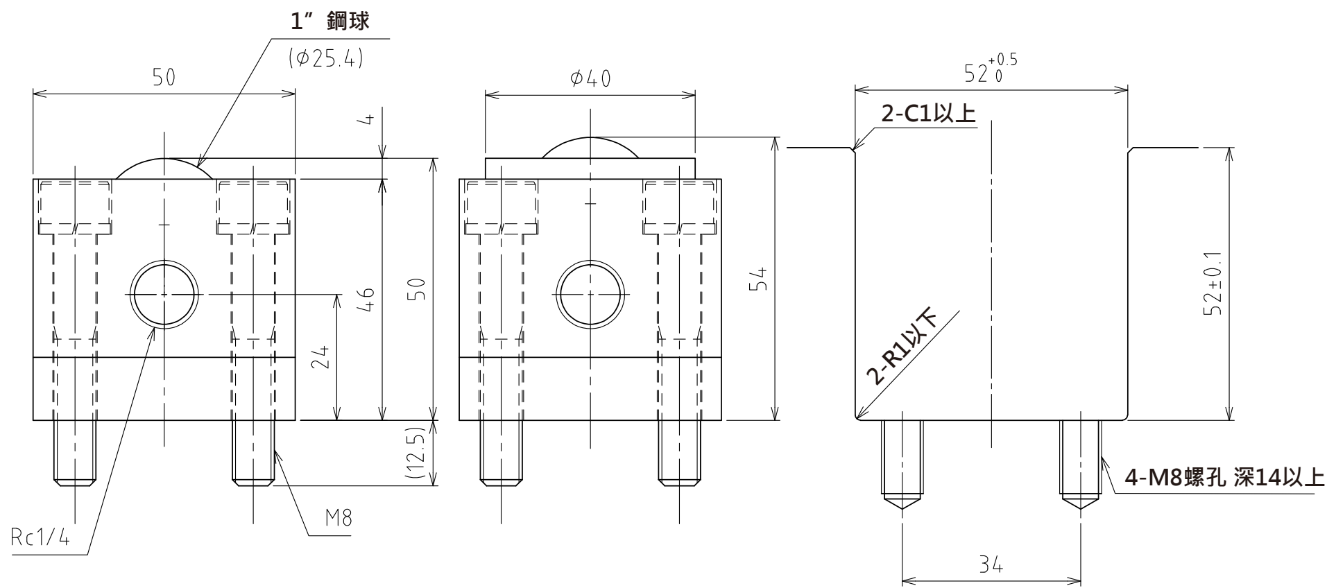
A視圖
