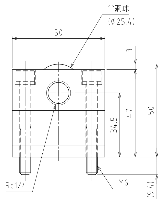
A視圖
