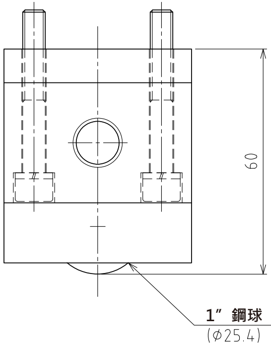
上浮時 (行程3mm)
