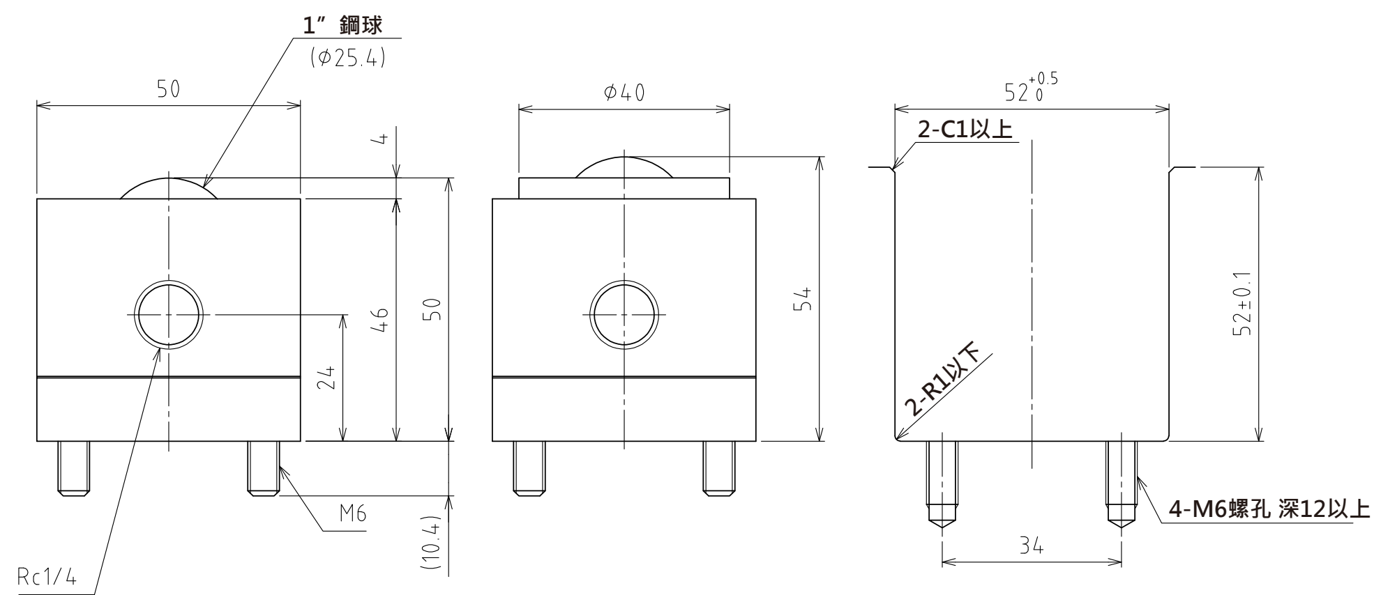
A視圖
