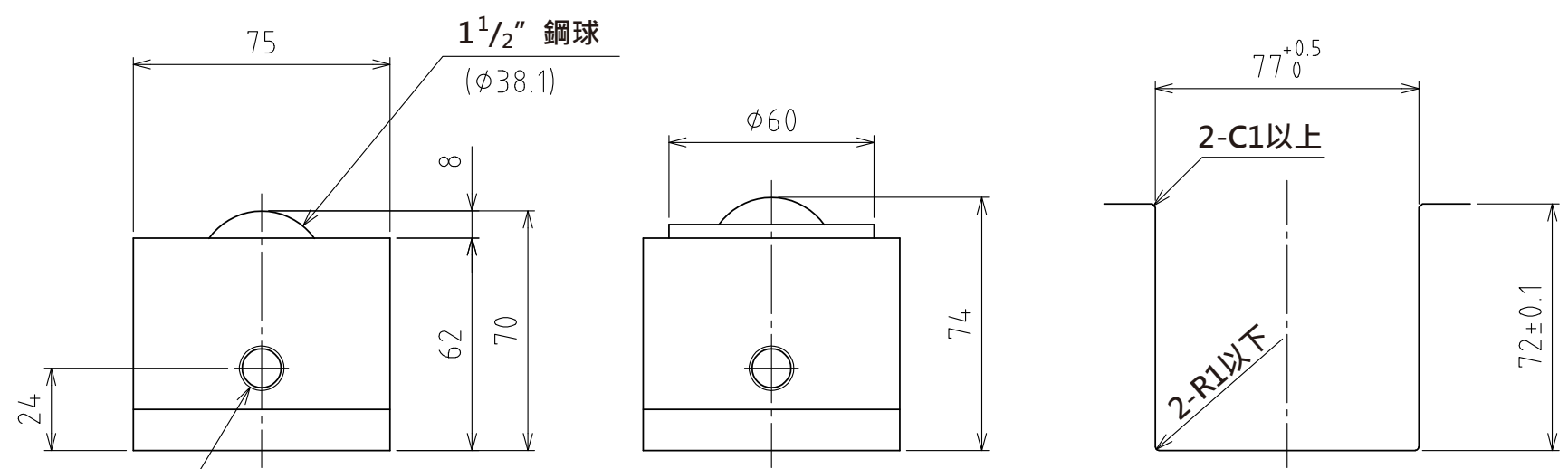
A視圖
