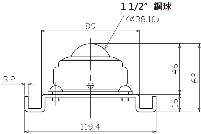
A視圖 (尺度 1 : 3)
