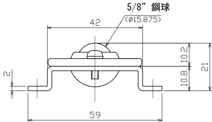
A視圖 (尺度 1 : 1)
