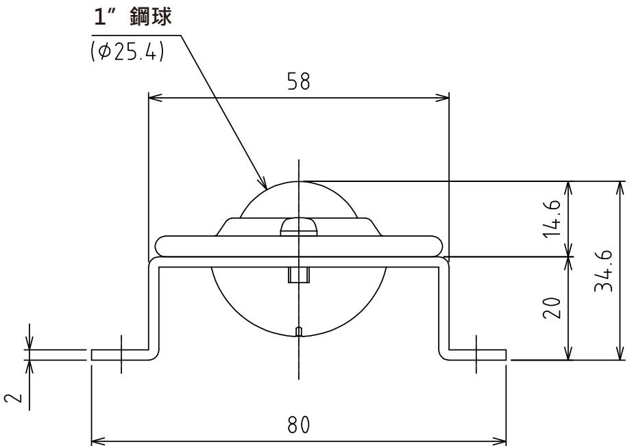
A視圖 (尺度 1:1)
